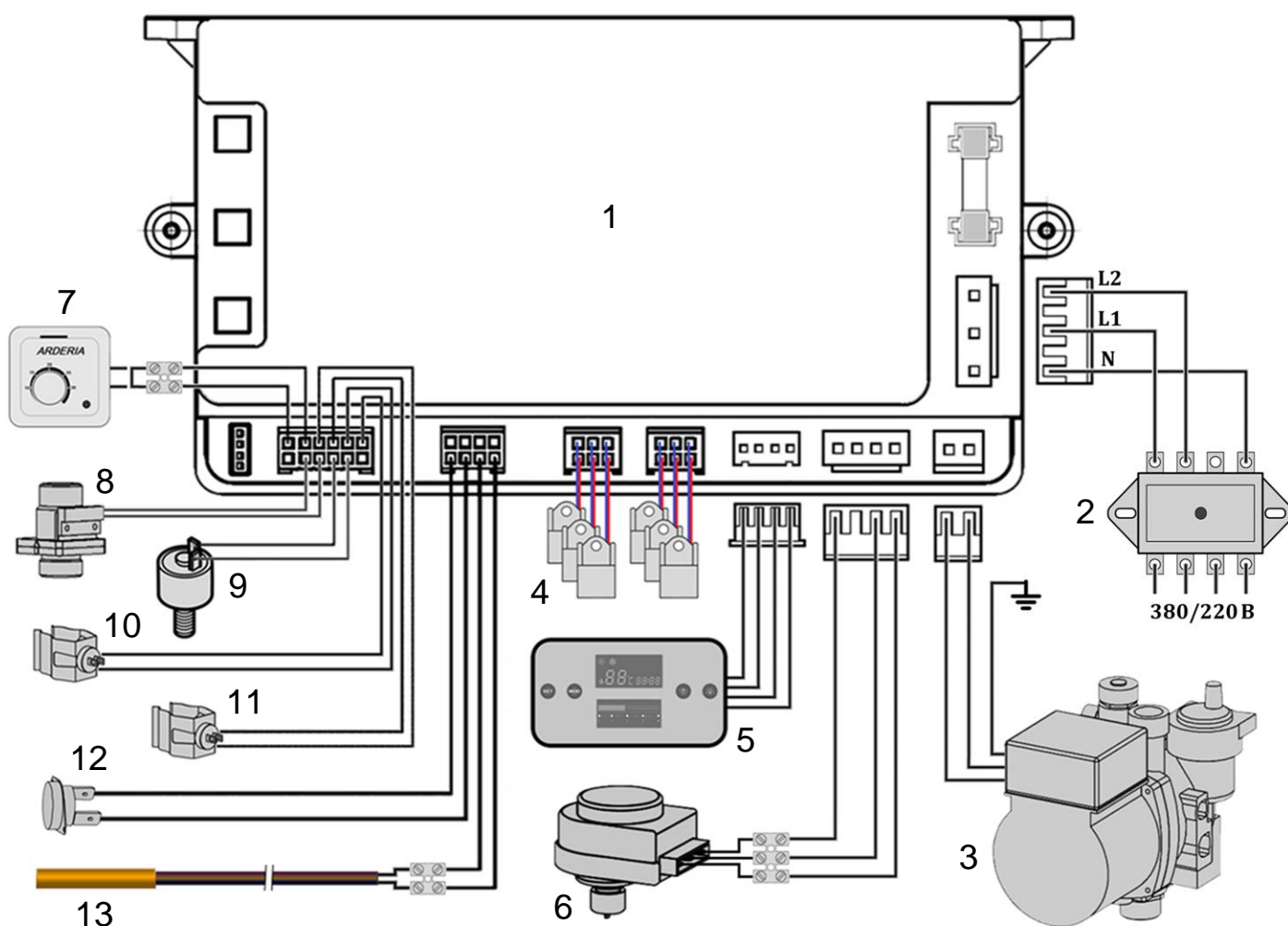
Рис.24 Принципиальная электрическая схема электрокотла Arderia
