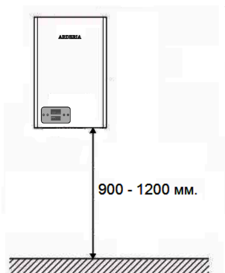
Рис. 10 Монтажные расстояния
