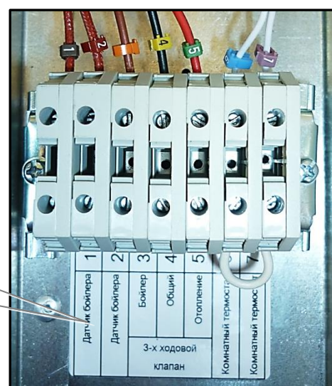
Рис.24 Подключение датчика температуры бойлера трёхходового клапана «ARDERIA» к клеммной колодке.
