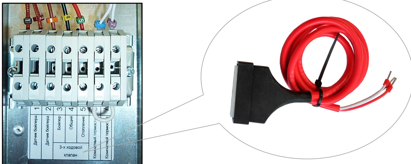
Рис.23 Подключение трёхходового клапана «ARDERIA» к клеммной колодке.
