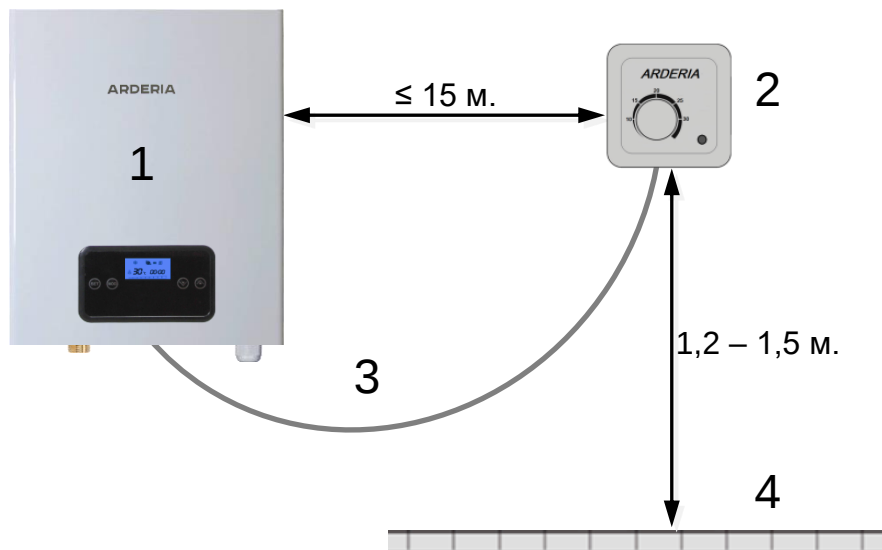
Рис. 21 Место установки комнатного термостата
