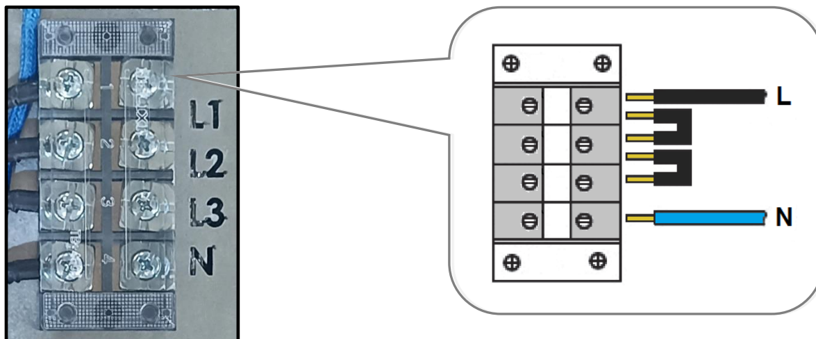
Рис. 11 Однофазное подключение
